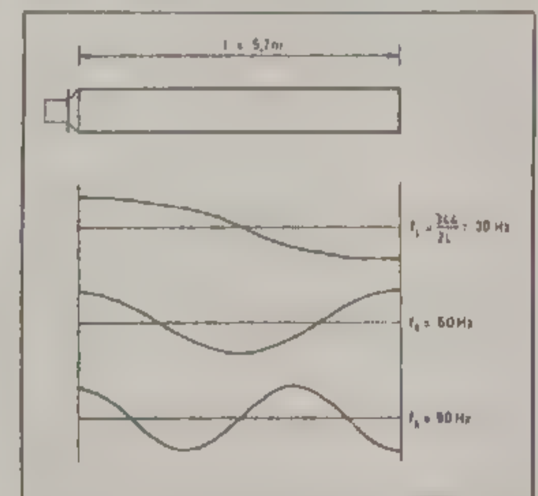
fig. 8 Eigenfrekwenties in een gesloten pijp.
